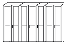
ŠATNÍ SKŘÍŇ, 7 DVEŘÍ TAKÉ VARIANTA SE 3 ZRCADLY š × v × h [mm] 3290 × 214 × 580
