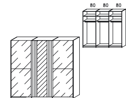
ŠATNÍ SKŘÍŇ, 5 DVEŘÍ, 3 ZRCADLA, 2 ZÁSUVKY š × v × h [mm] 2500 × 2230 × 640 přední plochy možné i varianta sklo
