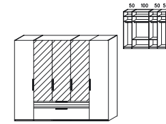
ŠATNÍ SKŘÍŇ, 5 DVEŘÍ, 3 ZRCADLA, 2 ZÁSUVKY š × v × h [mm] 2500 × 2230 × 640 přední plochy možné i varianta sklo
