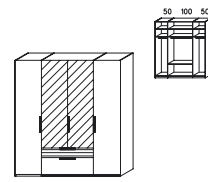
ŠATNÍ SKŘÍŇ, 4 DVEŘE, 2 ZRCADLA, 2 ZÁSUVKY š × v × h [mm] 2000 × 2230 × 640 přední plochy možné i varianta sklo
