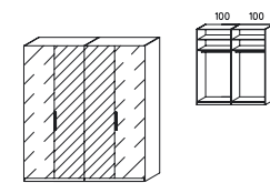
ŠATNÍ SKŘÍŇ, 4 DVEŘE, 2 ZRCADLA š × v × h [mm] 2000 × 2230 × 640 přední plochy sklo
