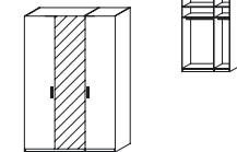
ŠATNÍ SKŘÍŇ, 3 DVEŘE, 1 ZRCADLO š × v × h [mm] 1510 × 2230 × 640
