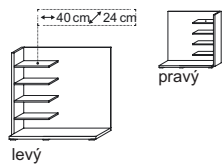
PŘÍDAVNÝ REGÁL KE KOMODĚ šíře komody 600mm š × v × h [mm] 1040 × 980 × 430
