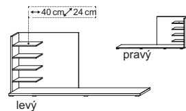
PŘÍDAVNÝ REGÁL KE KOMODĚ šíře komody 1800mm š × v × h [mm] 2240 × 980 × 430
