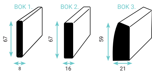
ROZMERY BOKOV
